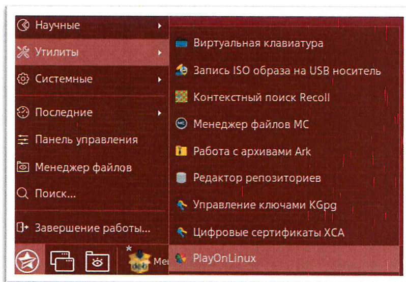
Рис 4. PlayOnLinux
